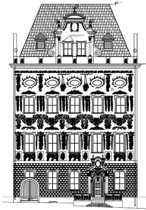
Rzut elewacji frontowej oraz przekrój A-A dla planowanej inwestycji.
